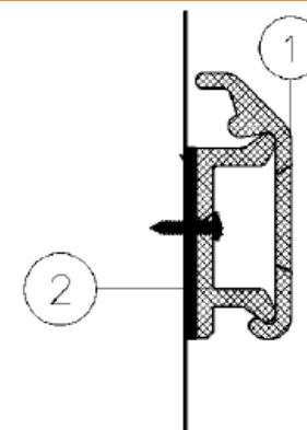
DETALLE DE MONTAJE ITEM 1 Y 2
